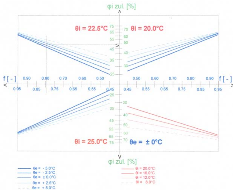
Bild 2: Zul. Raumluftfeuchte ( \phi_{i \text{ zul.}} ) je nach Temperaturfaktor ( f ) und Klima Zu Tabelle 1: Ablesung für d = 120 \text{ mm} : f_1 \sim 0.793 \rightarrow \phi_{i \text{ zul.}} \sim 48.3\%
